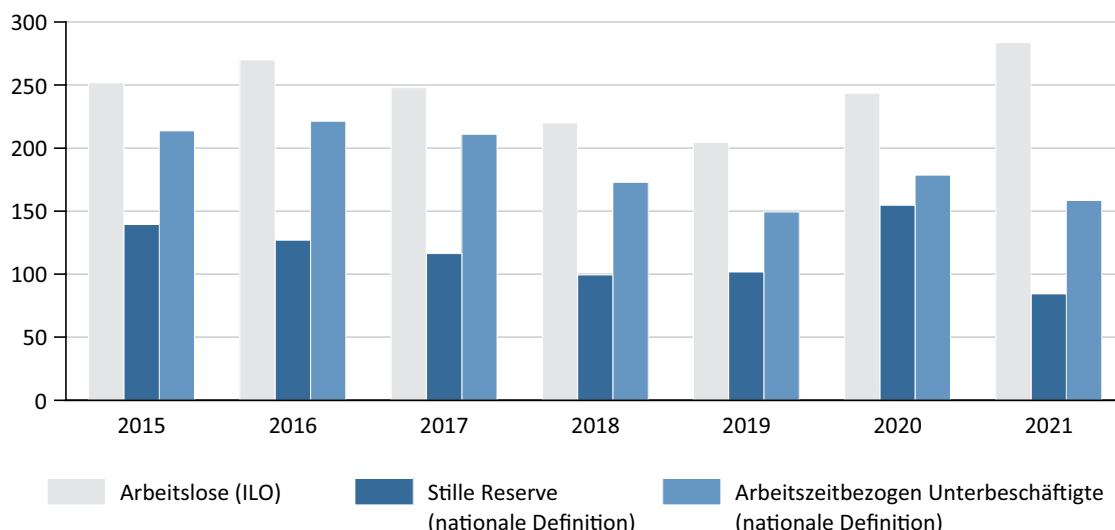
Grafik 6
