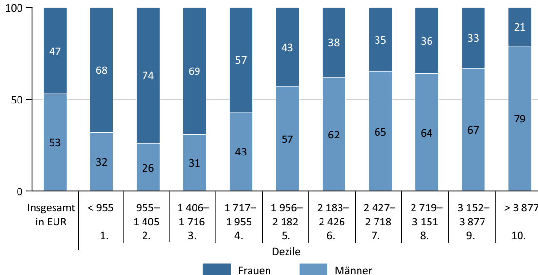
Grafik 7
