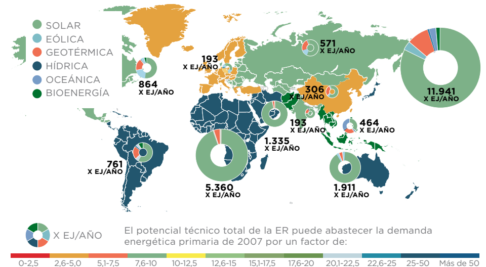
GRÁFICO 2 POTENCIAL TÉCNICO TOTAL DE LA ER EN EJ/AÑO PARA 2050 POR FUENTE DE ENERGÍA RENOVABLE
