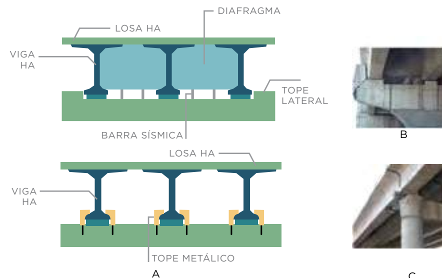
GRÁFICO 3 MODIFICACIONES ESTRUCTURALES AL DISEÑO DE PUENTES PREVIO AL 27-F
