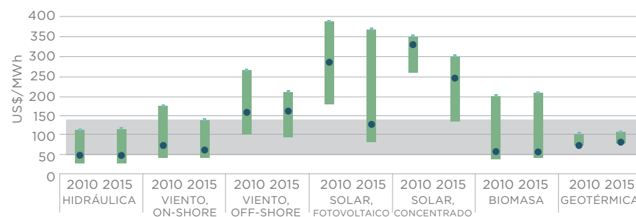
GRÁFICO 4 COSTOS NIVELADOS POR TECNOLOGÍA (PROMEDIO PONDERADO GLOBAL Y RANGOS)
