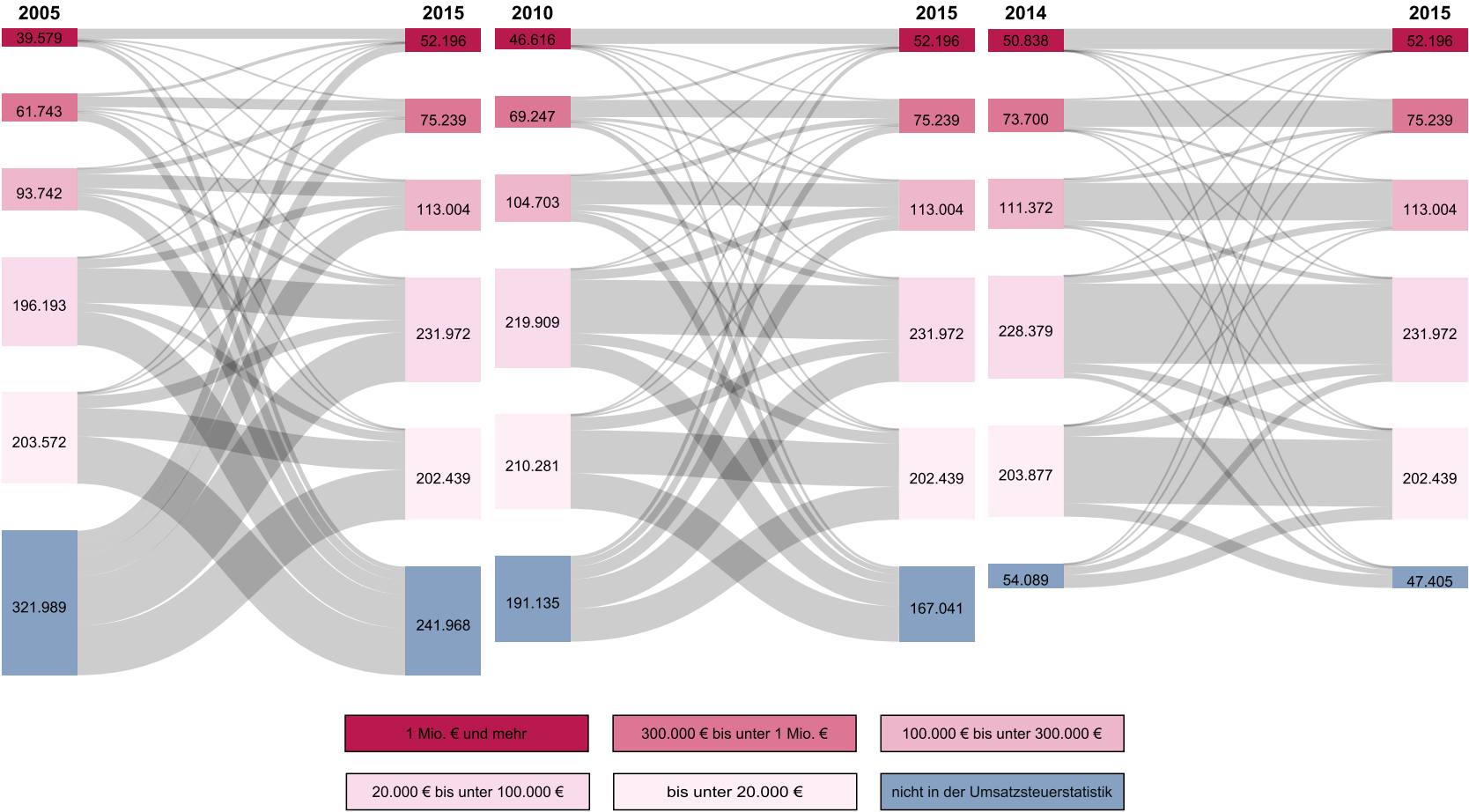
Grafik 2 Verteilung der Umsatzsteuerfälle nach Stufen des steuerbaren Umsatzes in Jahresvergleichen zwischen 2005 und 2015, 2010 und 2015 sowie 2014 und 2015
