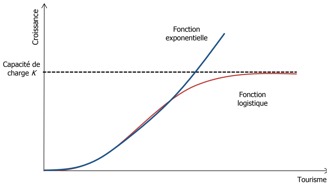
Figure 31 : Représentation d'une fonction exponentielle et d'une fonction logistique
