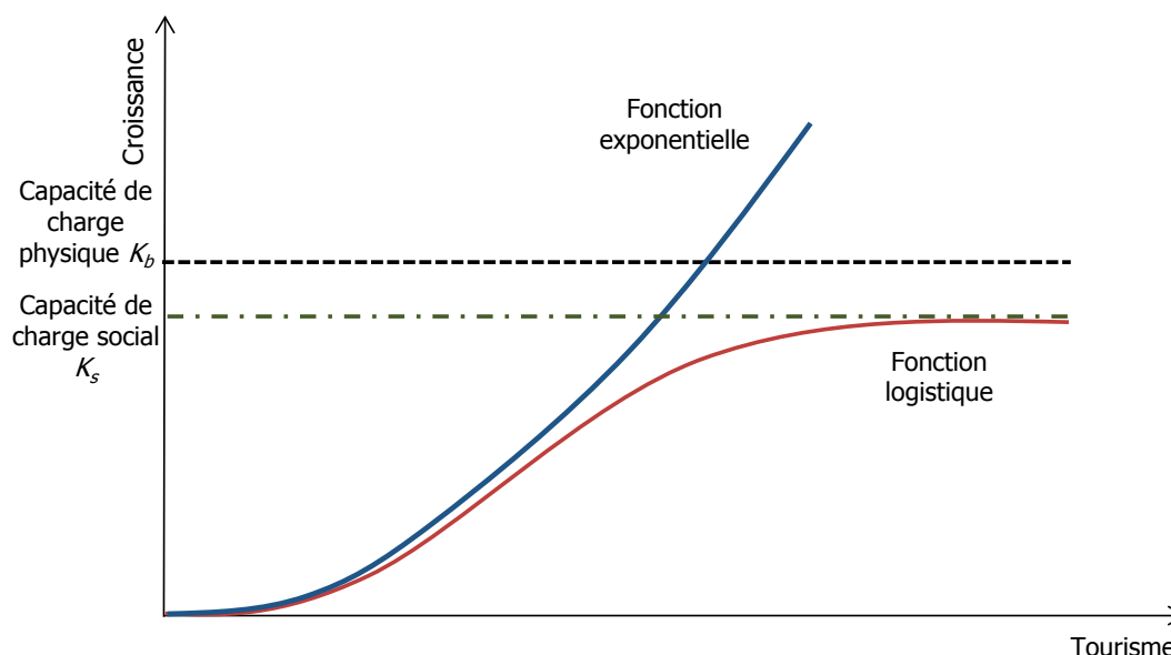
Figure 33 : Représentation d'une fonction exponentielle et d'une fonction logistique
