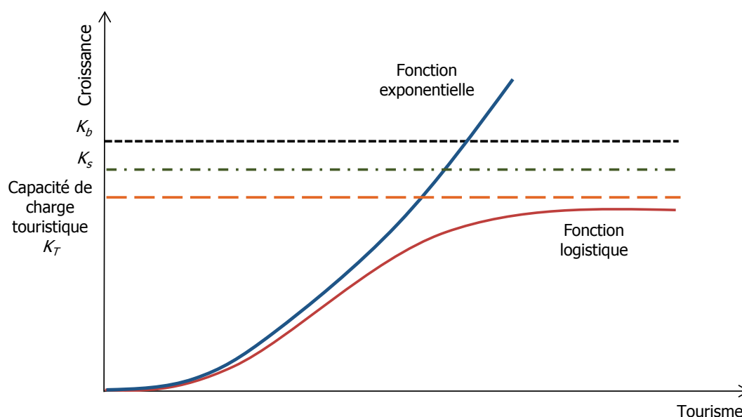
Figure 34 : Représentation d'une fonction exponentielle et d'une fonction logistique
