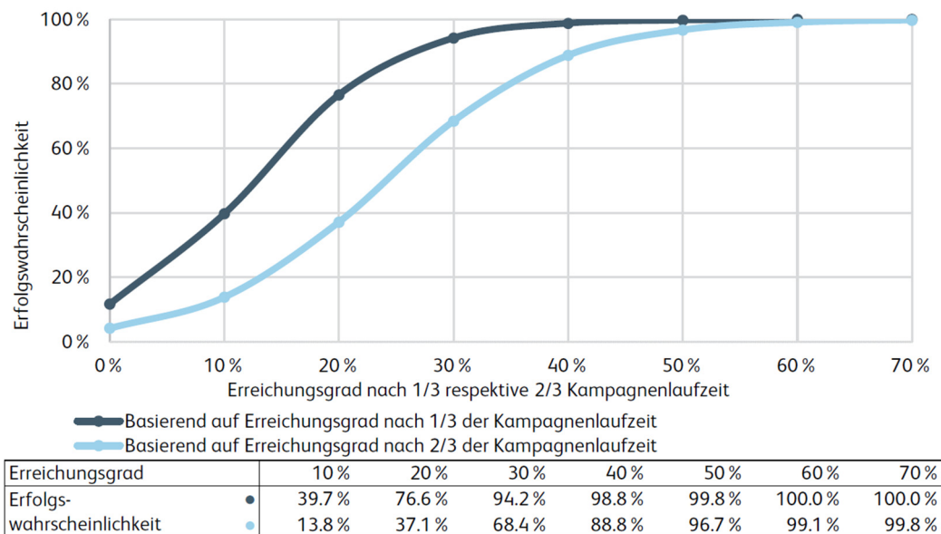
Abbildung 11: Prognostizierte Erfolgswahrscheinlichkeit
