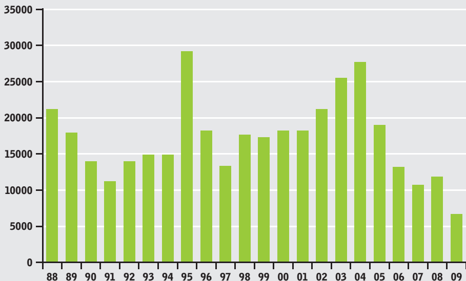
Abbildung 1: Legale Entwaldungsraten in Amazonien in km 2 pro Jahr
