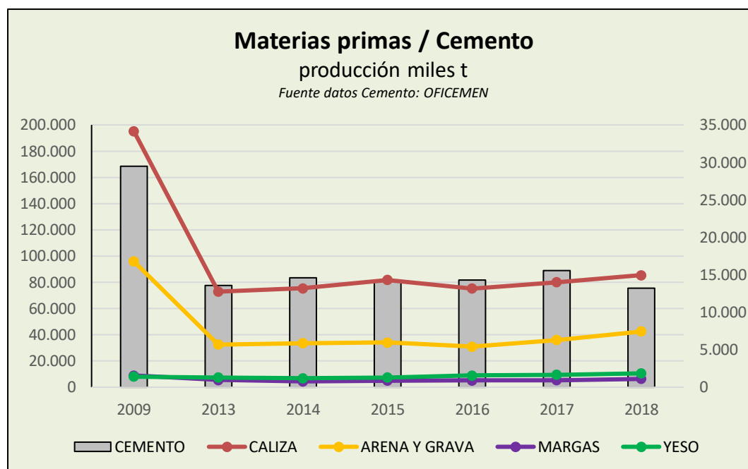
Gráfico 5 – Comparativa materias primas / cemento
