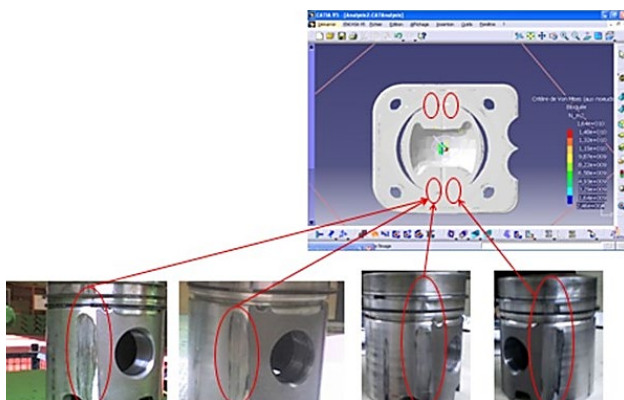
Fig. 2. Seizure piston
