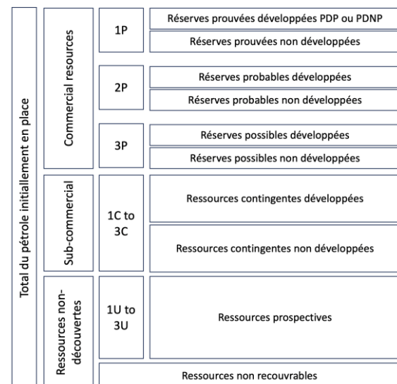
Figure 1 : Classification des réserves, schéma simplifié
