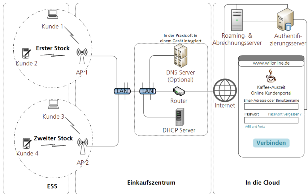
Abb. 05 Aufbau eines öffentlichen WLAN-Netztes, bestehend aus Authentifizierungsserver, Einstiegsseite und mehreren APs, um eine größere Fläche abdecken zu können. Die Abbildung zeigt die Verbindung der APs über LAN.
